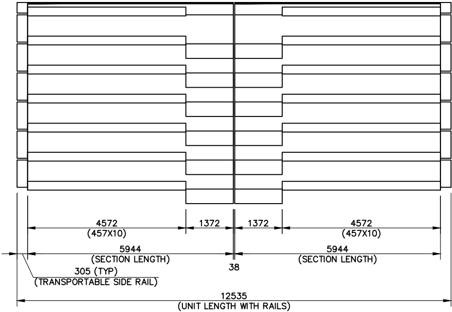
BANK E2 70 (PORTABLE)
