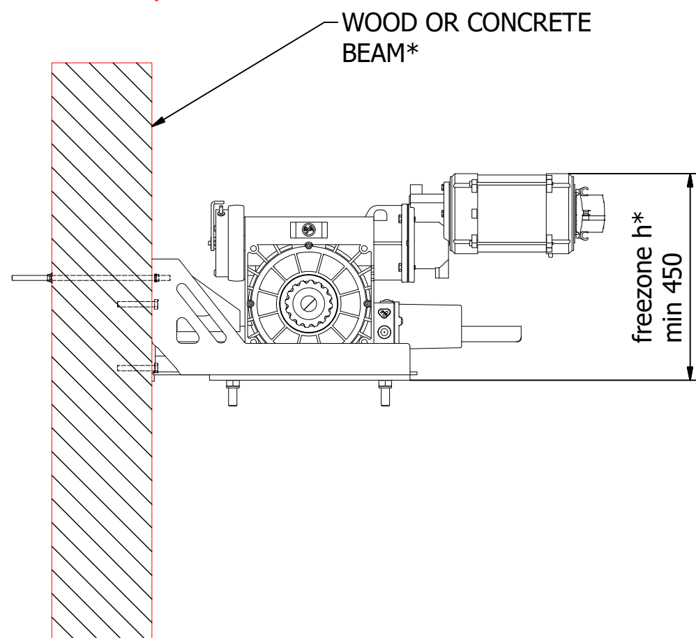
SECTION D-D
